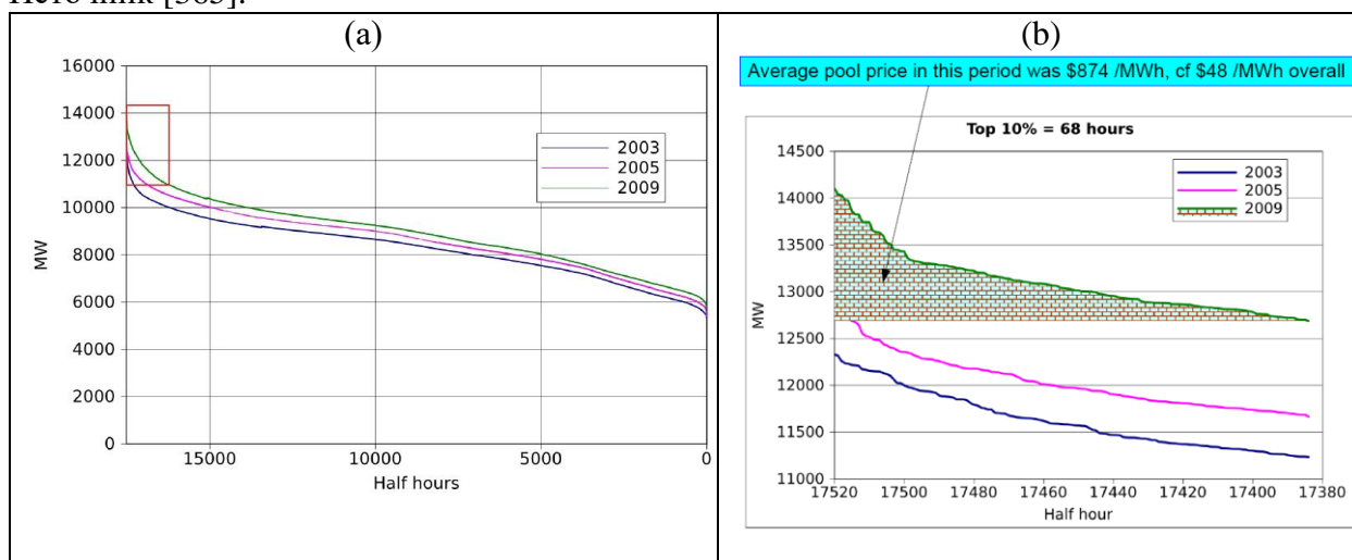
Рис. 3. Годовой график получасовых нагрузок Нового Южного Уэльса (NSW Австралия), (время (получасовые интервалы); нагрузка (МВт)).
