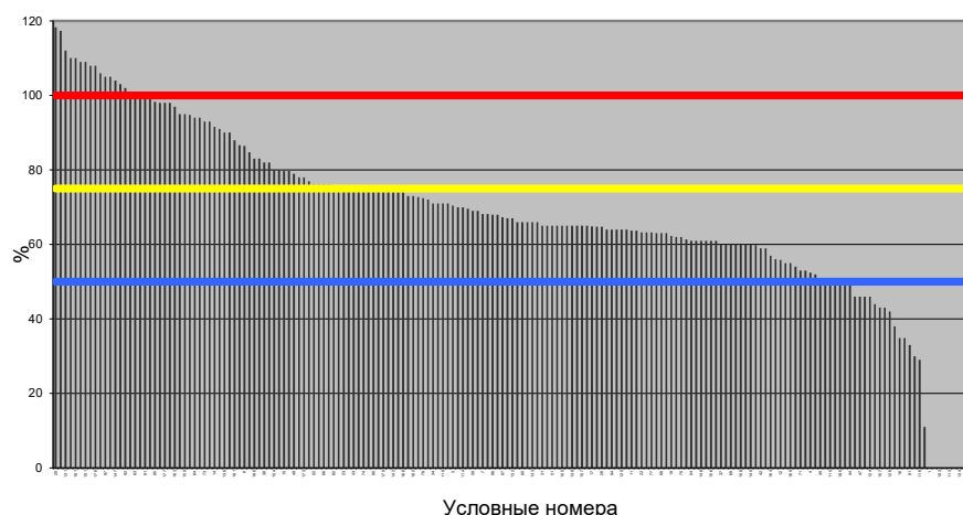
Загрузка трансформаторов ПС 110кВ 15.12.2004г.
